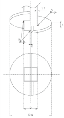
先端翼の形状 (軸部：角型鋼管)
